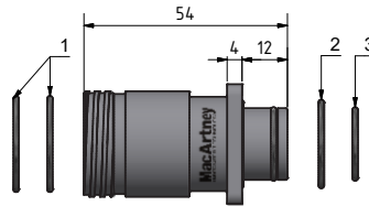
TrustLink Metal Shell FCR SA
